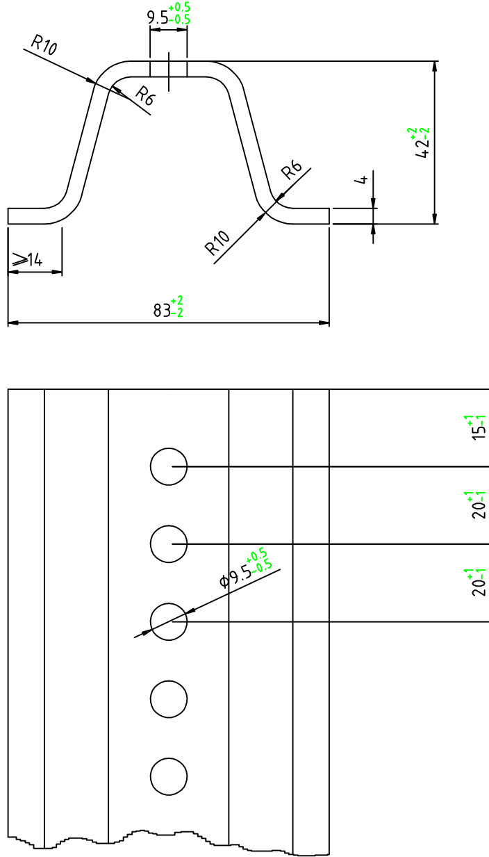
ŞEKİL 2: 4 mm kalınlığındaki omega profil için şekil ve ölçüler.
